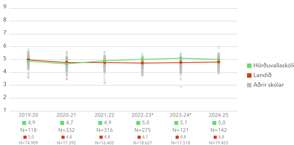
3.1. Samsömun við nemendahópinn – Ársmeðaltöl
