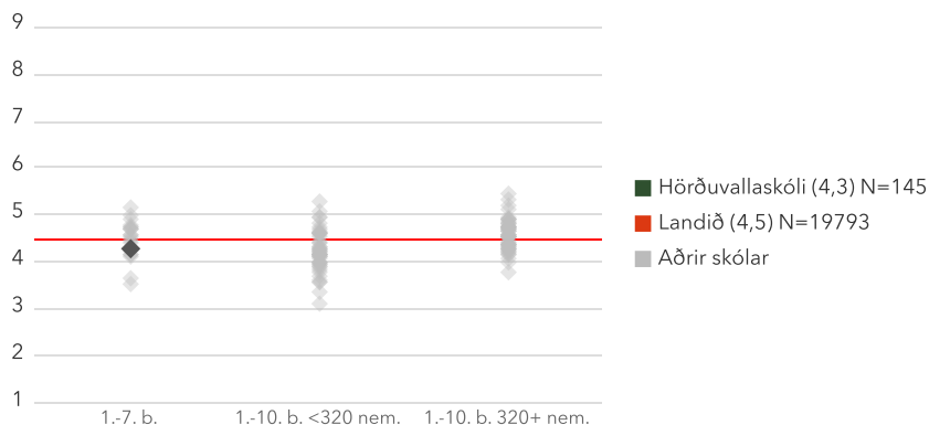
1.2. Þrautseigja í námi – Röðun
