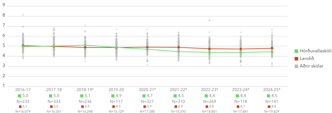
3.3. Agi í tímum – Ársmeðaltöl
